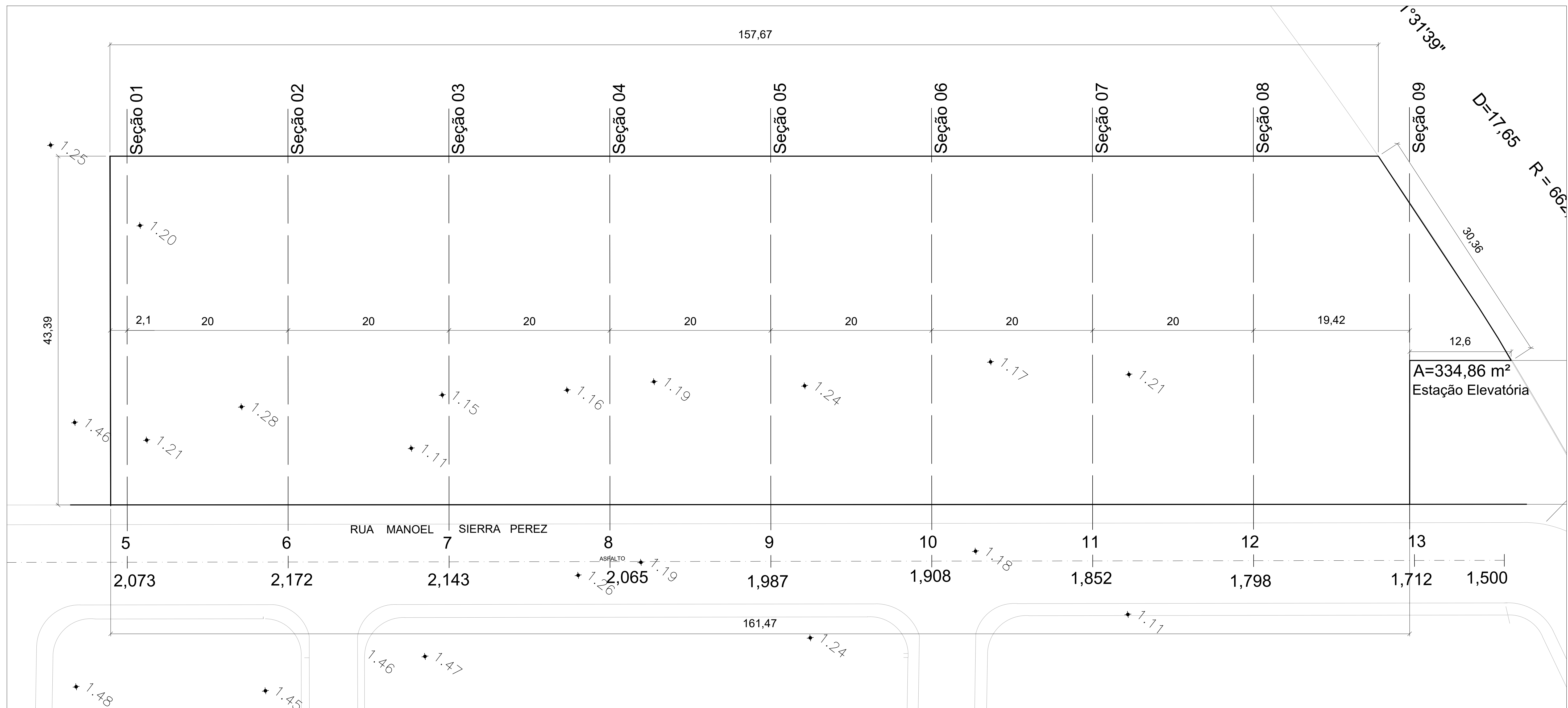
ÁREA INSTITUCIONAL - I-1 Esc.: 1/250
